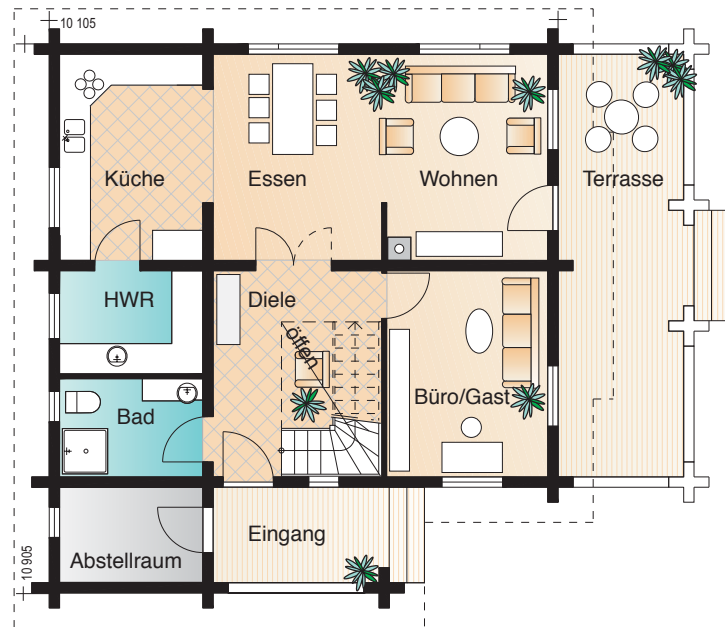
Erdgeschoß 1:150
