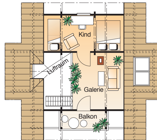
Dachgeschoß 1:150
